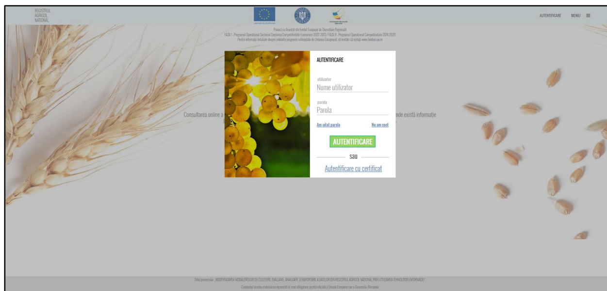
Fig. 36 Accesare portal
