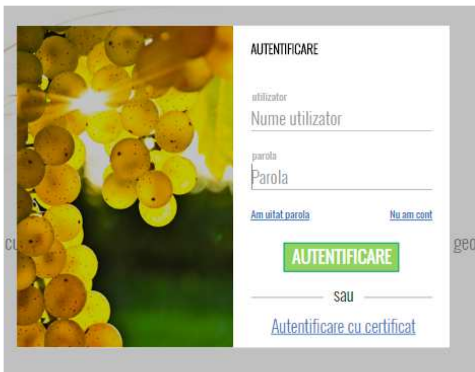
Fig. 8 Ecran autentificare
